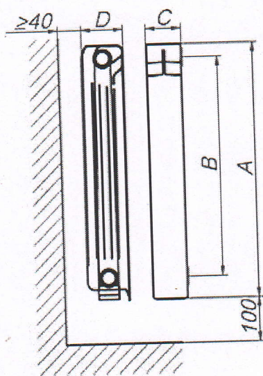
Ugradnja na otvoreni ravni zid
